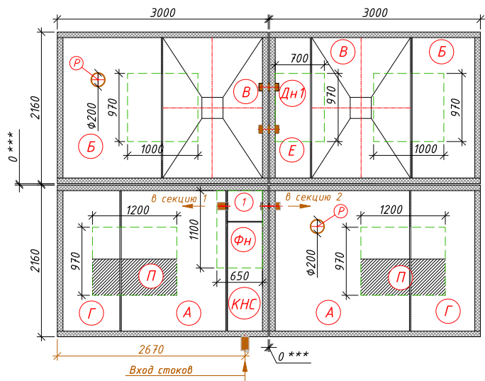
Схема станции
